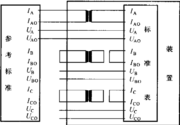
图 C2 相间交变磁场影响试验状态
