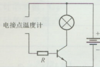
图 2 信号电路
